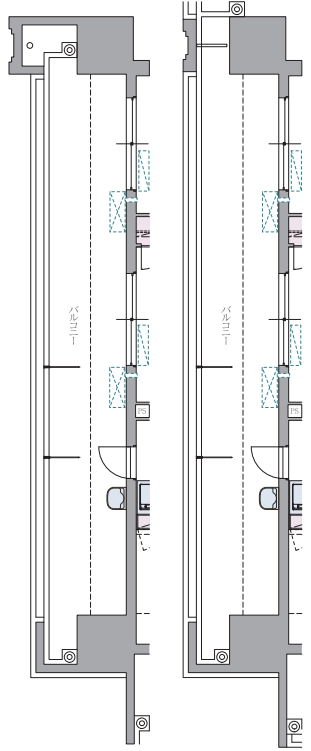
2階バルコニー 部分図(E1) scale ≒ 1/150
