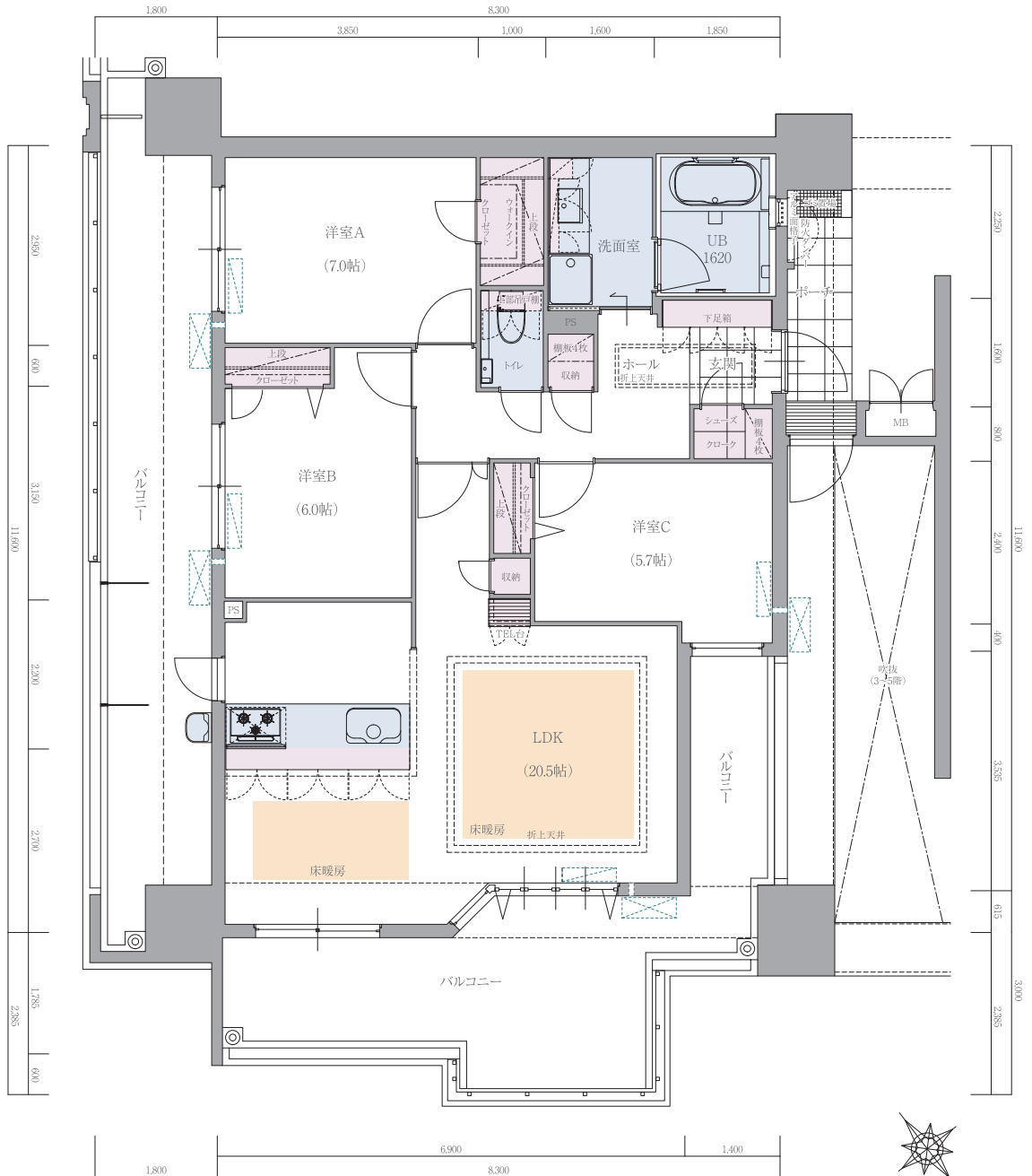
3階バルコニー 部分図(E) scale ≒ 1/150
